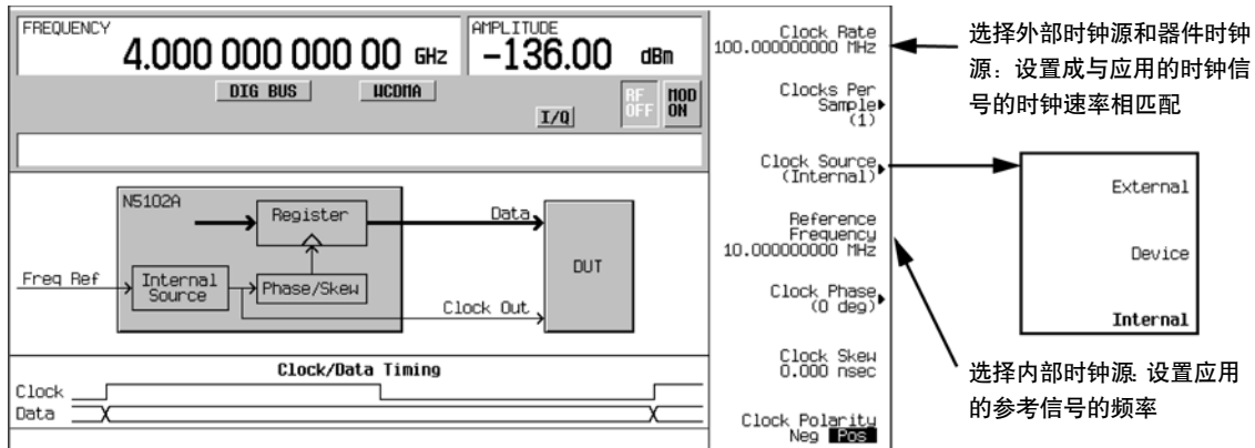
图 11-2 时钟源选择
