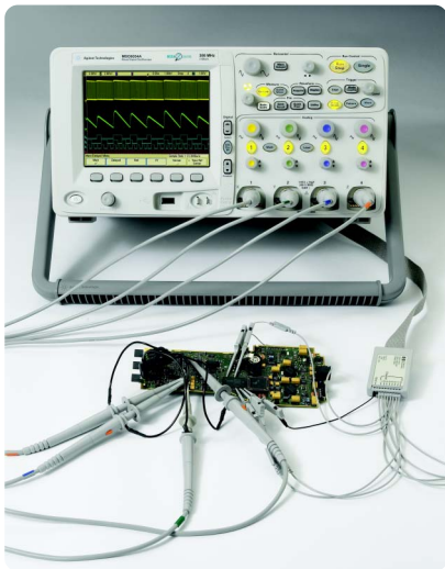
图 2. 4+16 通道 MSO 使您能用一台仪器观察 4 个模拟信号和 16 个数字信号。
