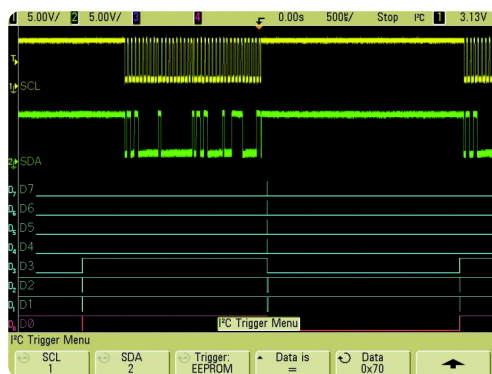
图 11. 在 I 2 C 帧内的地址和 / 或数据码型上触发
