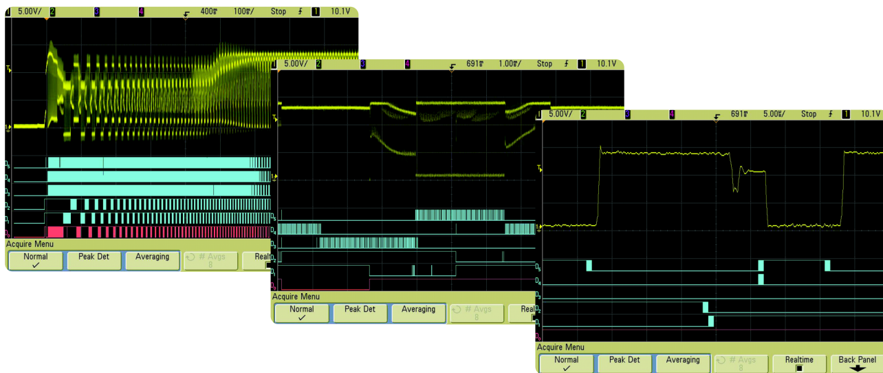
图 3. 使用数字控制信号触发的马达驱动信号起动序列，用 Agilent MSO6000A 系列 MSO 的不同倍数放大揭示“矮”脉冲。
