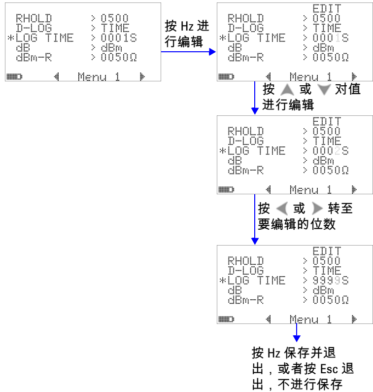
图 4-4 “interval (time) logging” 的记录时间设置
