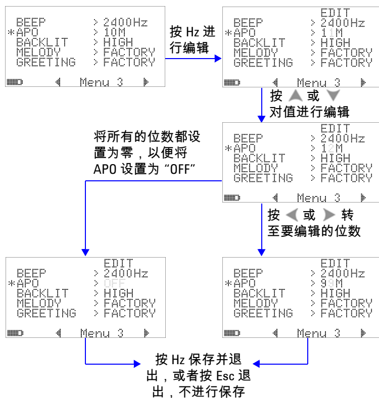
图 4-13 自动节能设置
