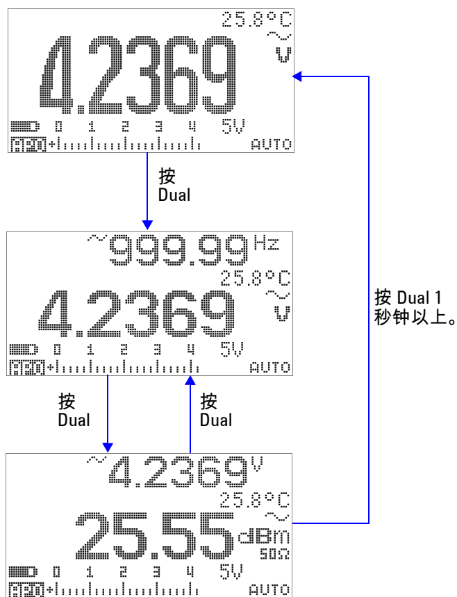
图 3-5 dBm 显示模式下的操作
