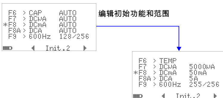
图 4-28 编辑初始测量功能 / 范围和初始输出值
