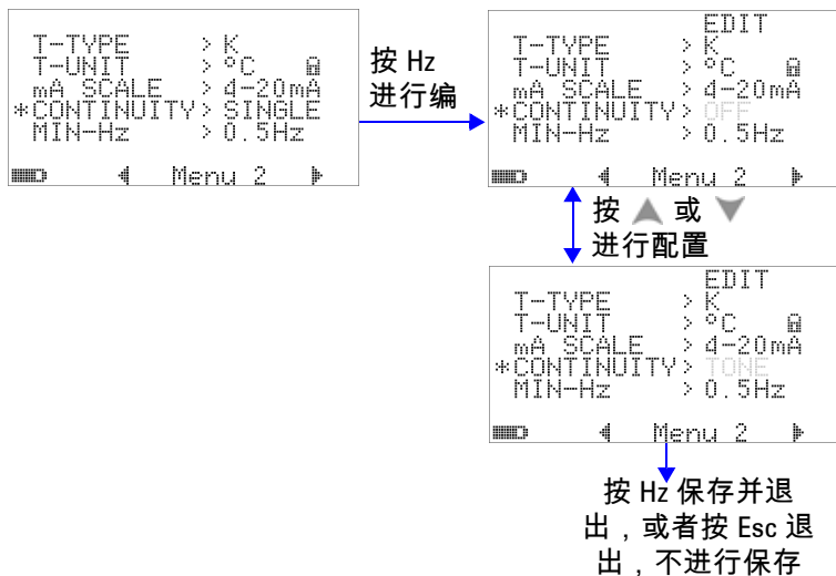
图 4-10 选择通断测试中所使用的声音
