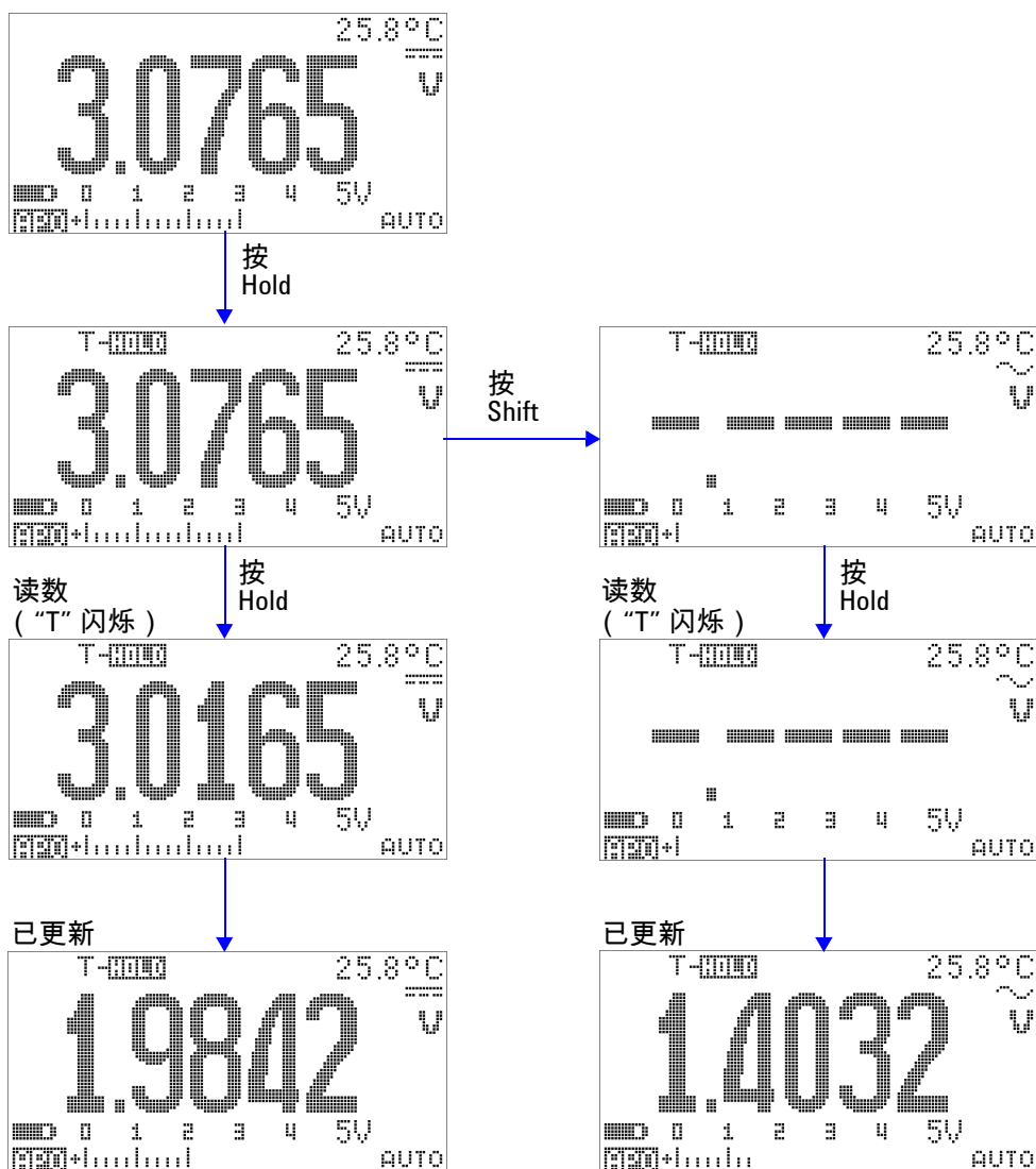
图 3-2 “Data hold” 模式下的操作
