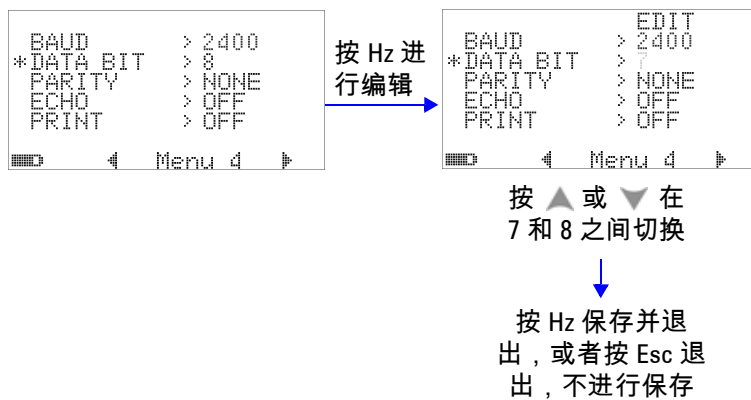
图 4-19 远程控制的数据位设置
