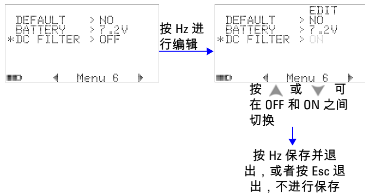
图 4-32 DC 滤波器
