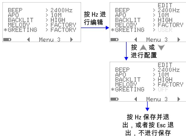
图 4-16 电源打开时的问候语设置
