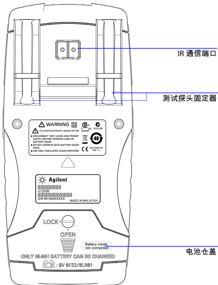
图 1-6 U1253B 的后面板
