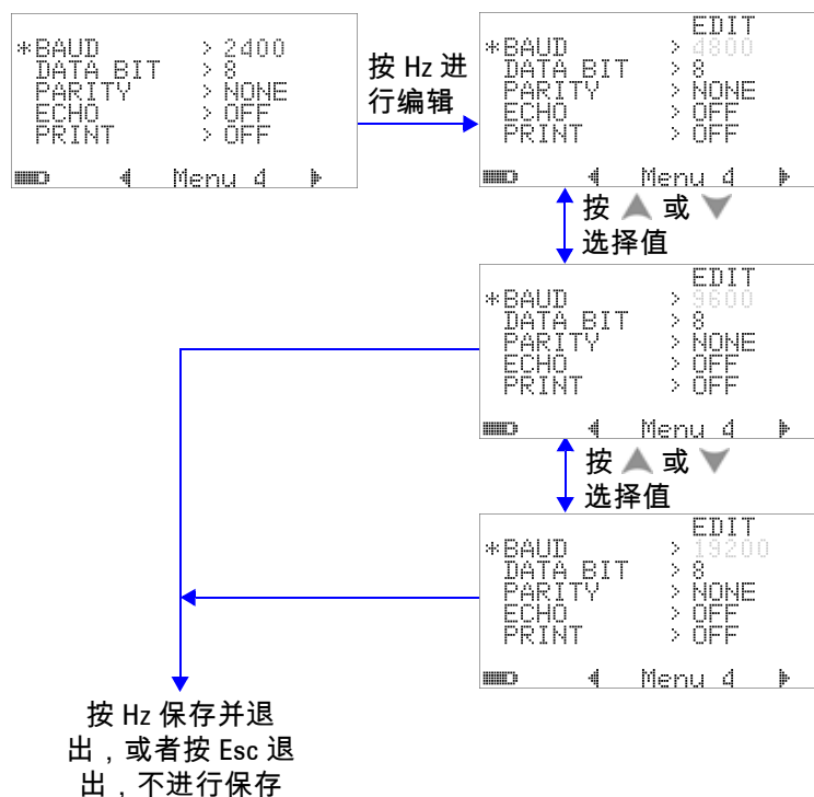
图 4-17 远程控制的波特率设置
