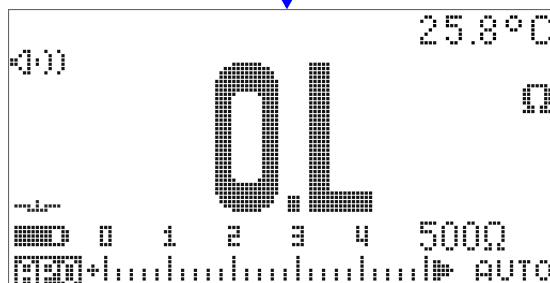
图 2-10 短路通断和断路通断测试
