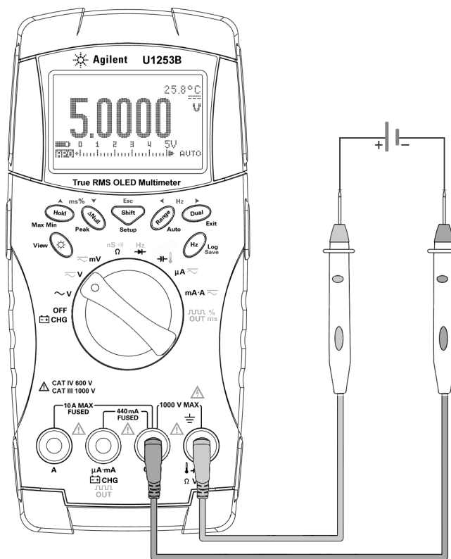
图 2-2 测量 DC 电压
