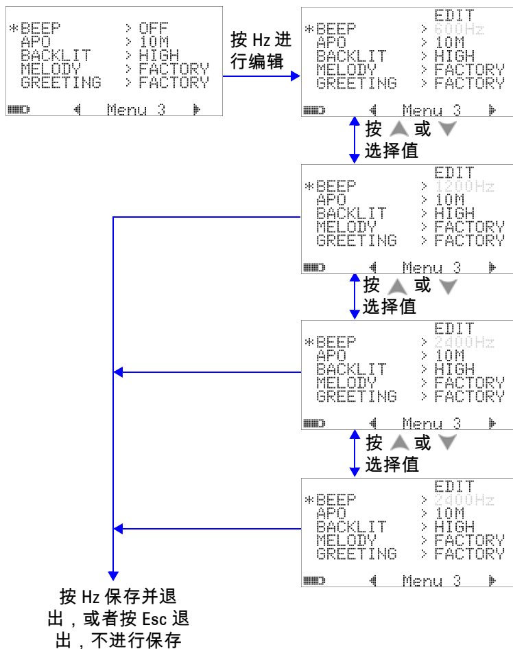
图 4-12 蜂鸣声频率的设置
