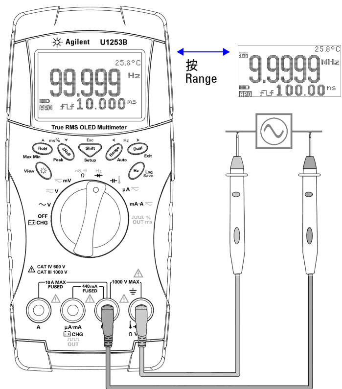
图 2-6 测量频率
