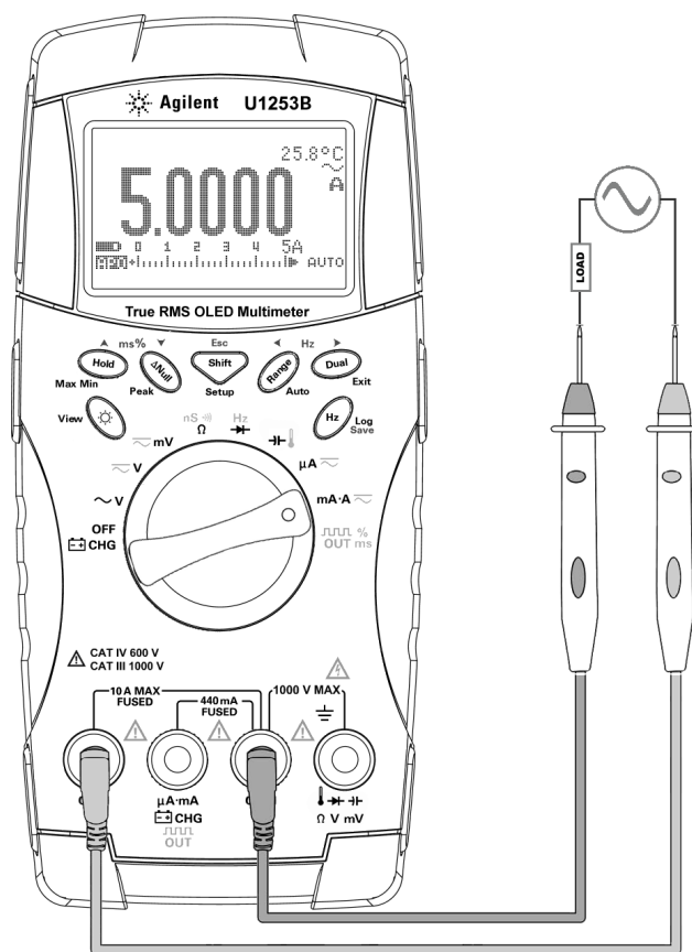
图 2-5 A (安培) 电流测量
