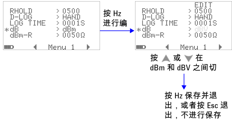
图 4-5 分贝测量设置
