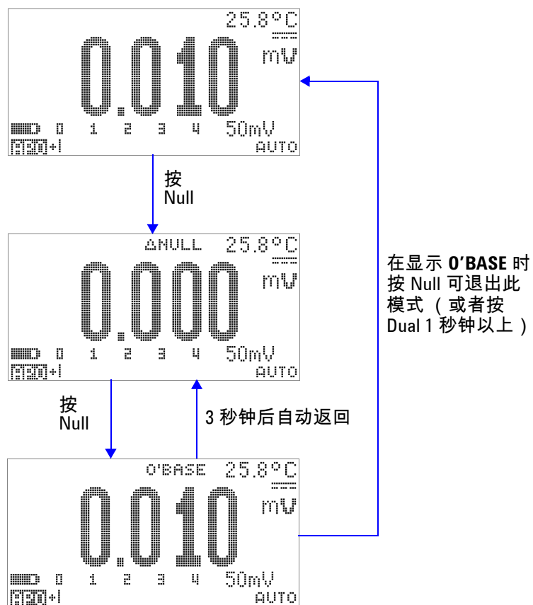
图 3-4 “Null” ( 相对 ) 模式下的操作
