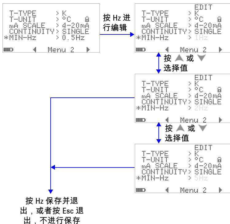
图 4-11 最小频率的设置
