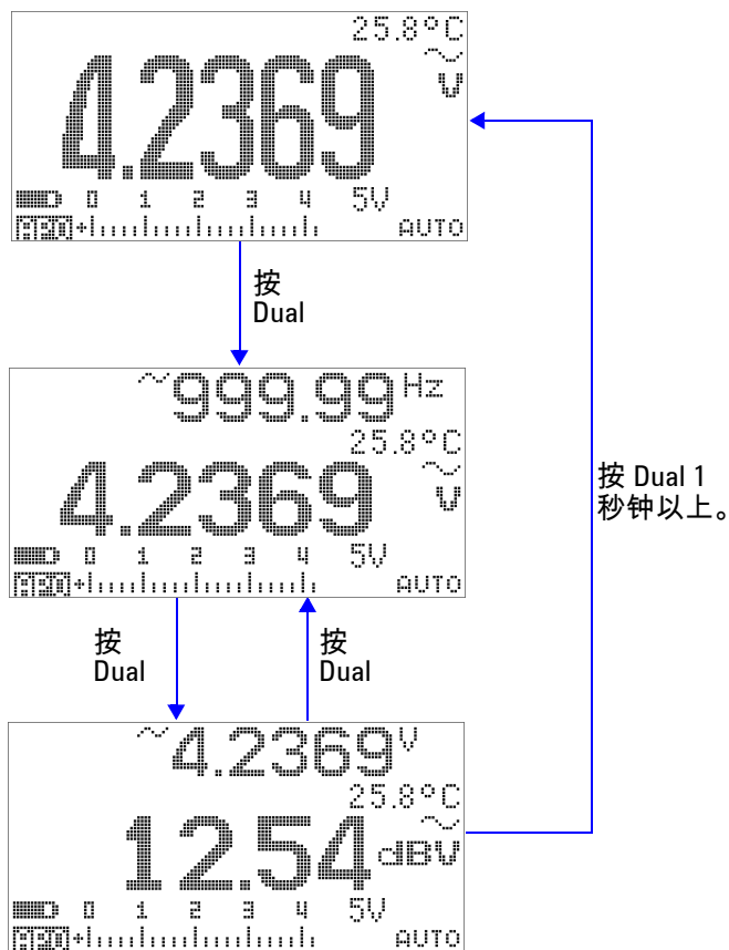
图 3-6 dBV 显示模式下的操作
