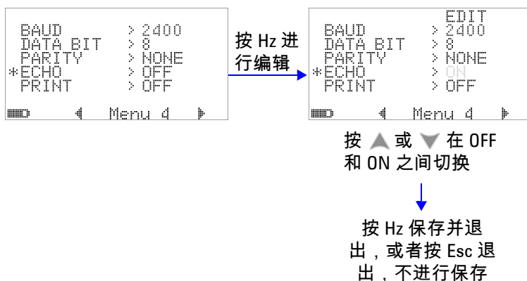
图 4-20 远程控制的回波模式设置
