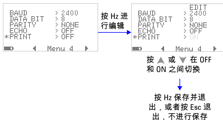
图 4-21 远程控制的打印模式设置
