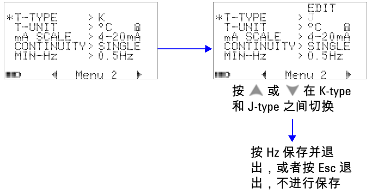
图 4-7 热电偶类型设置
