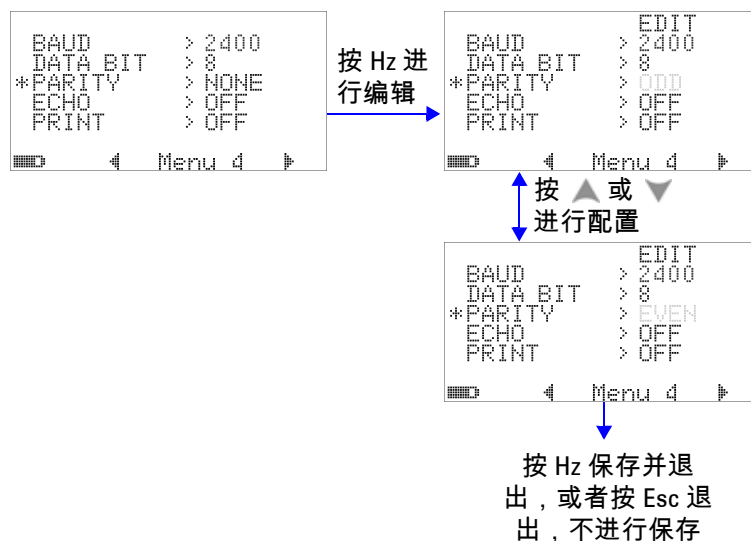
图 4-18 远程控制的奇偶校验设置
