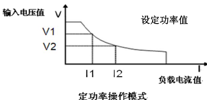
图 4-4 定功率模式电压电流图
