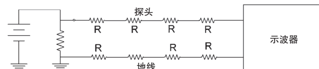
a. DC (0 Hz) 信号的分布式电阻
