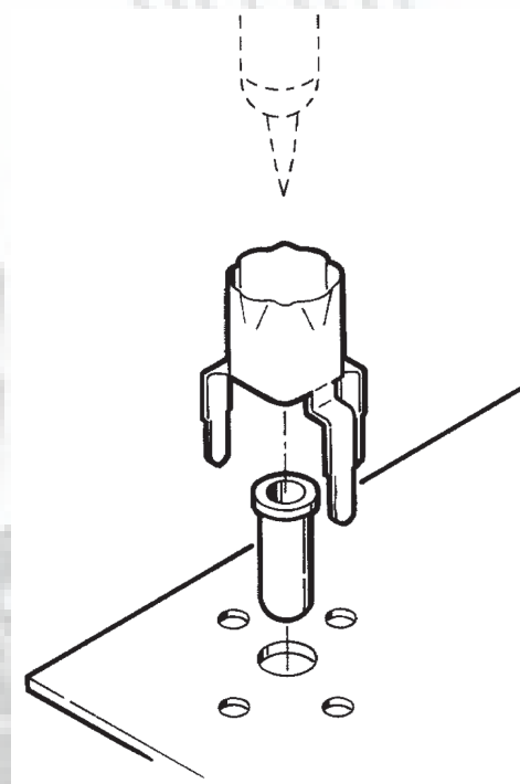
图 6.2. ECB 到探头尖端适配器。
