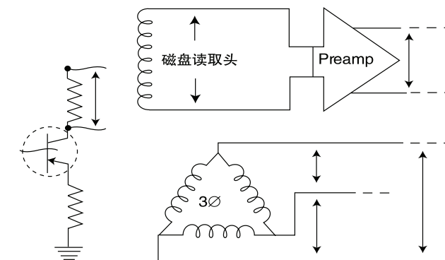
图 2.3. 部分差分信号源实例。
