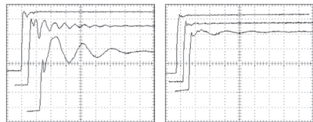
图 6.4. 无源探头与有源探头相比地线影响的实例。左面的三条轨迹显示了在无源探头上使用 1/2 英寸、6 英寸和 12 英寸地线时对波形的影响。右面的轨迹显示了使用同一条地线采集的同一波形，但使用的是有源 FET 探头。
