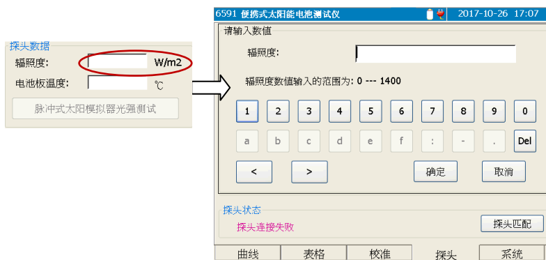
图 5-23 辐照度数值编辑示意图
