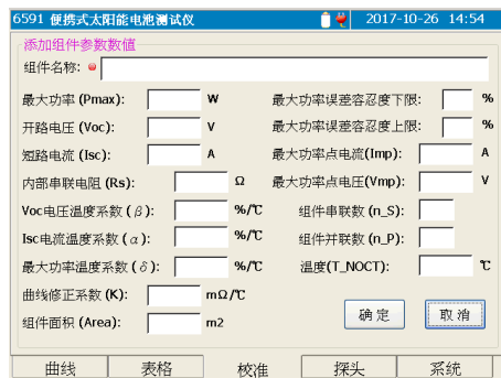
图 5-16 添加组件参数示意图
