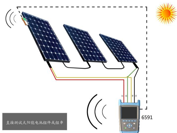
图 4-8 直接测试太阳能电池组串示意图
