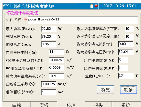
图 5-18 组件参数修改
