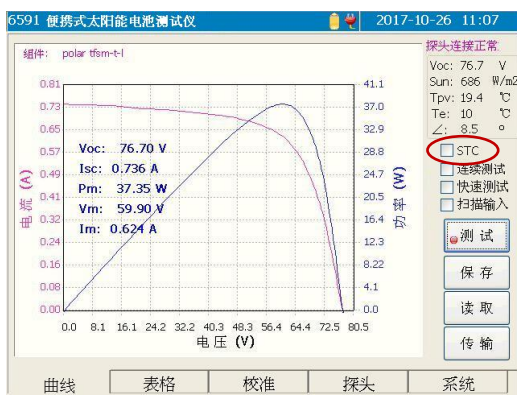
当前测试条件下的原始测试曲线
