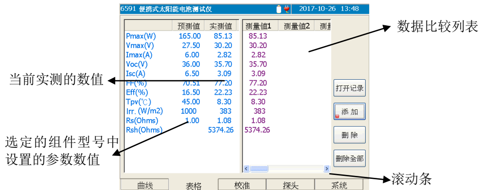
图 5-10 表格窗口示意图
