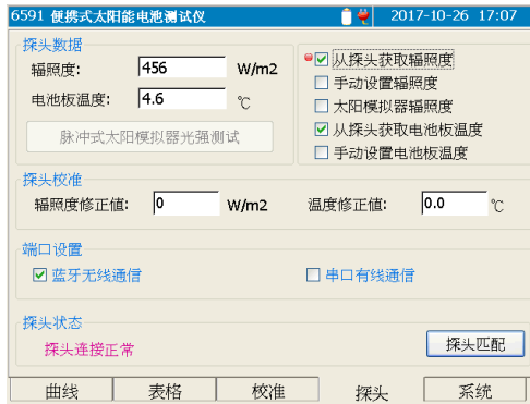
图 5-20 辐照度计窗口示意图
