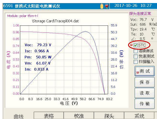
转换为 STC 下的测试曲线
