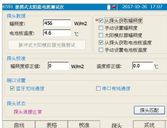
图 4-10 辐照度计窗口示意图
