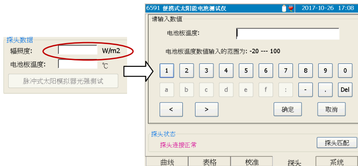
图 5-24 数值编辑框示意图
