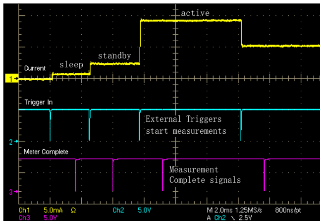
图2 器件上电时对启动负载电流进行测量
