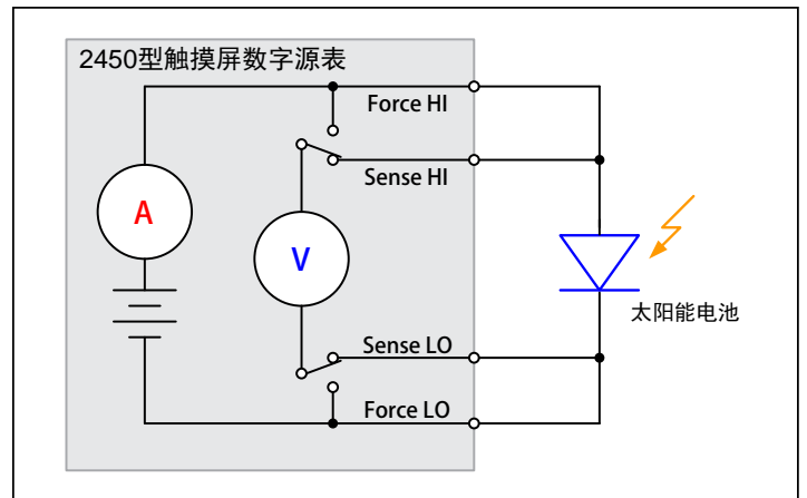
图5 太阳能电池与2450型仪器连接示意图
