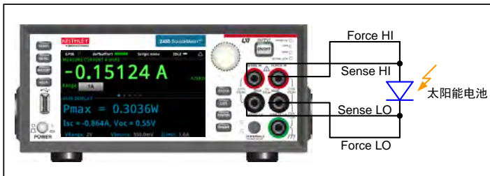
图1 2450型触摸屏数字源表与太阳能电池的连接
