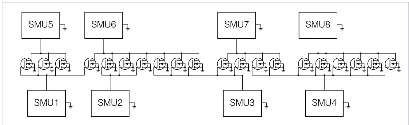
使用 8 个 SMU 对 20 个器件进行并行 HCI 和 NBTI 测试的实例。公共端子使用单独的接地单元 (GNDU)。
