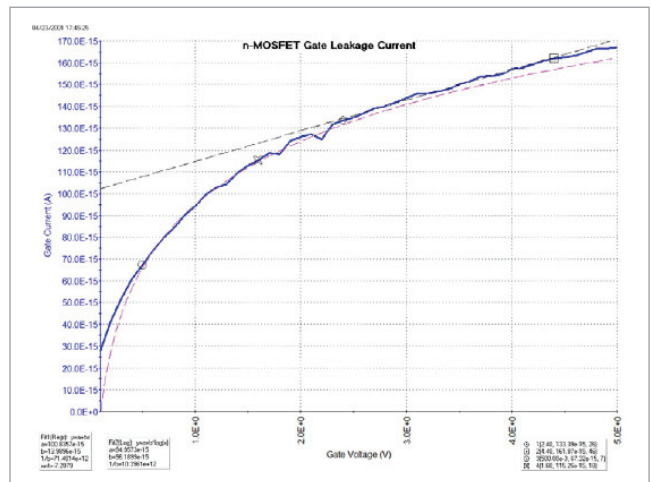
选配 4200-PA 前端放大器模块，fA 级测量。
