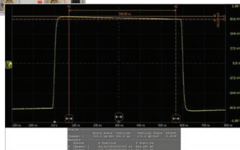
MOST150 SP2 一致性测试眼图
