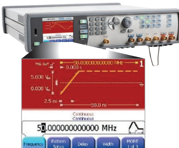
81160A 脉冲函数任意噪声发生器
