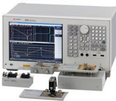
采用 E5061B ENA 系列网络分析仪进行网络和阻抗组合分析
