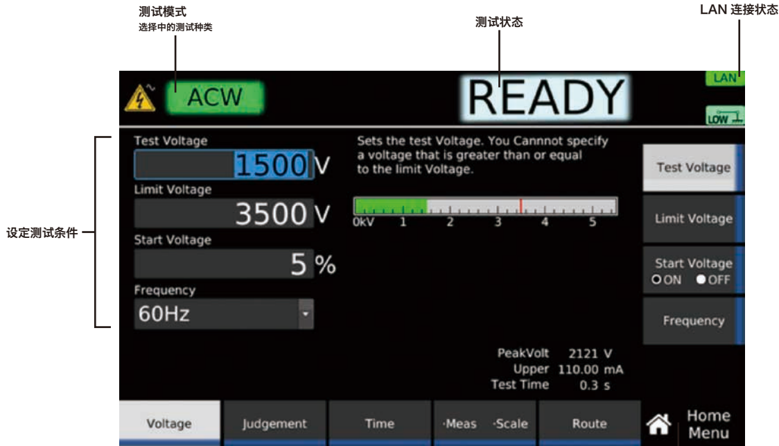
▲ Home Menu 画面 设定各种测试的测试条件以及执行测试。
