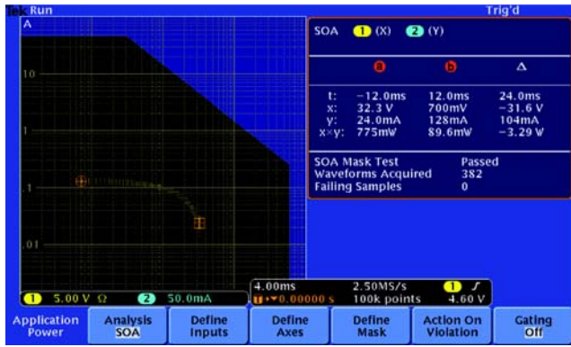
安全工作区测量。自动电源测量功能可以迅速准确地分析常用电源参数。
