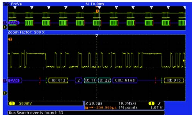
搜索步骤 2: Wave Inspector 自动搜索和记录每个事件, 并用空心白三角标记事件。然后可以使用 Previous 和 Next 按钮, 从一个事件跳到下一个事件。
