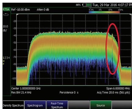
图 5. RTSA 能够以“密度显示”模式显示测量结果，在指定的频率扫宽上提供信号命中功能。此功能使其能够利用独特的统计功能，更容易地识别含有功率电平波动的两个不同信号。此屏幕快照显示了 RTSA 如何快速清晰地看到“威胁”。
